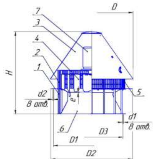
Габаритные и присоединительные размеры
