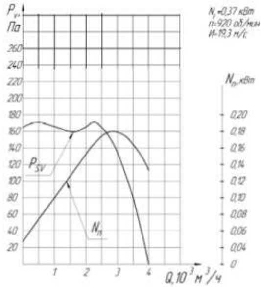
Рисунок 2 – Аэродинамические характеристики ВКР-4
