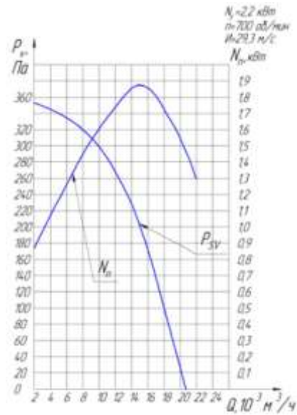
Рисунок 5– Аэродинамические характеристики ВКР-8
