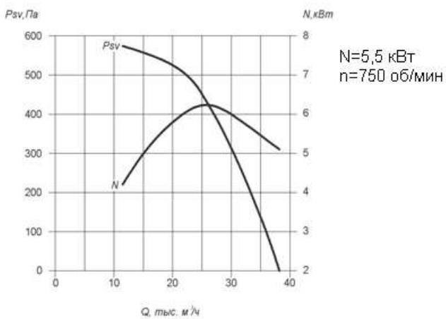
Рисунок 6– Аэродинамические характеристики ВКР-10
