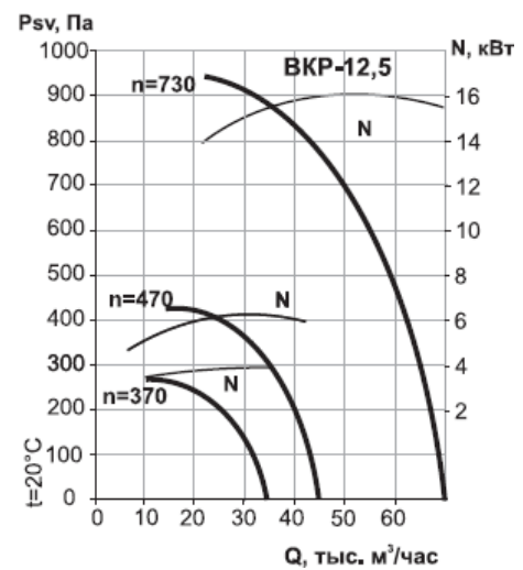
Рисунок 7– Аэродинамические характеристики ВКРМ-12,5
