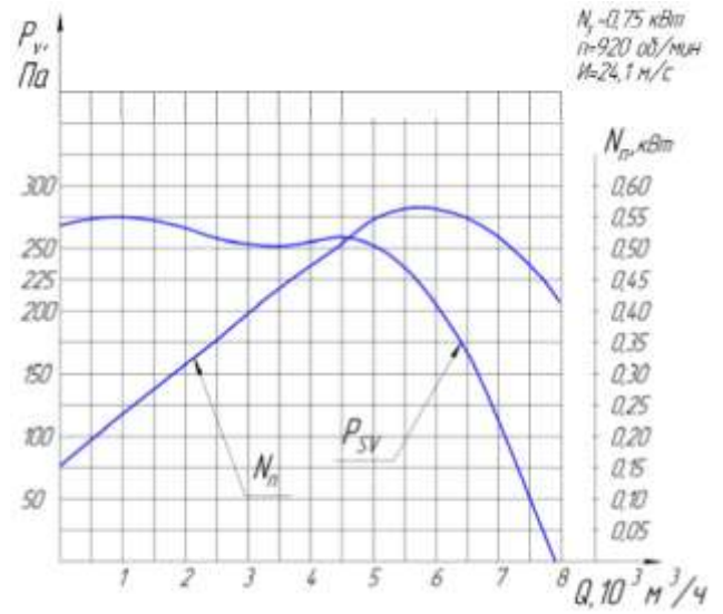
Рисунок 3 – Аэродинамические характеристики ВКР-5
