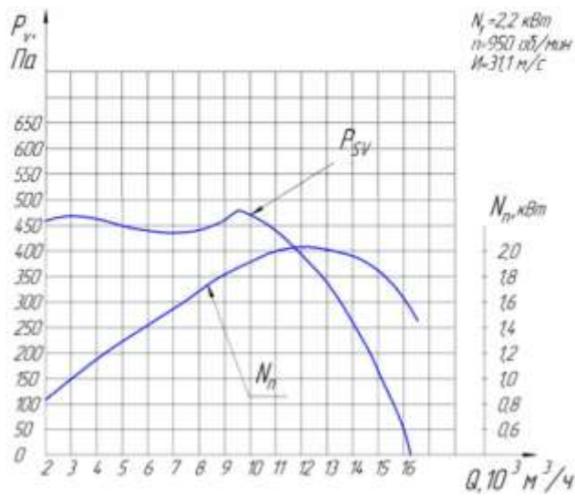
Рисунок 4– Аэродинамические характеристики ВКР-6,3
